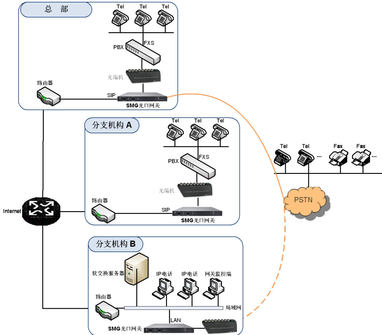
图 1-1 SMG 光口网关应用场景图
