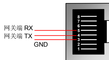
图 1-8 串口信号定义
