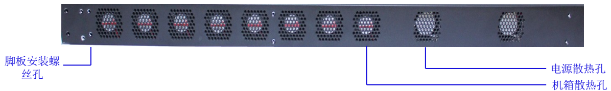
图 1-7 SBC2000 左侧示意图
