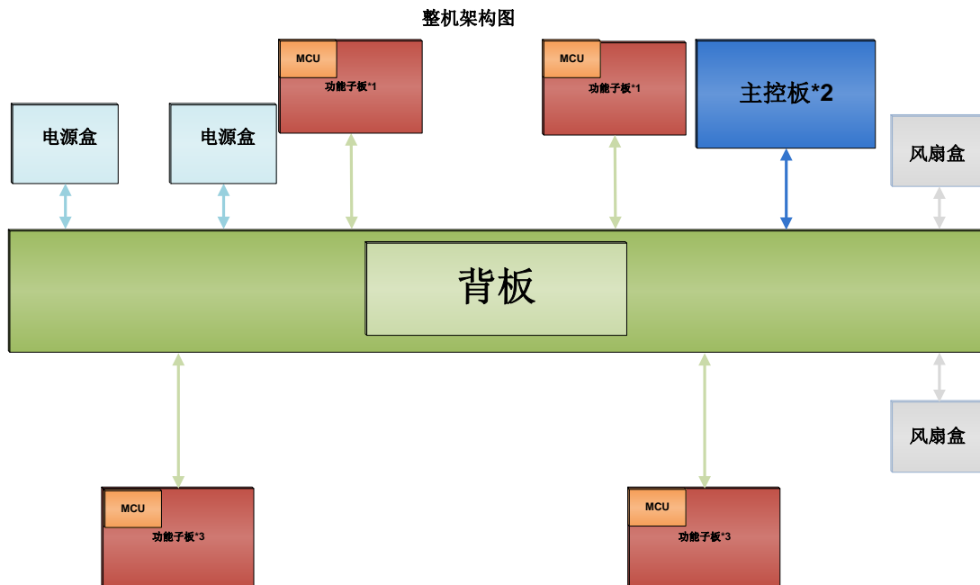
图 1-5 UMG 网关硬件架构图
