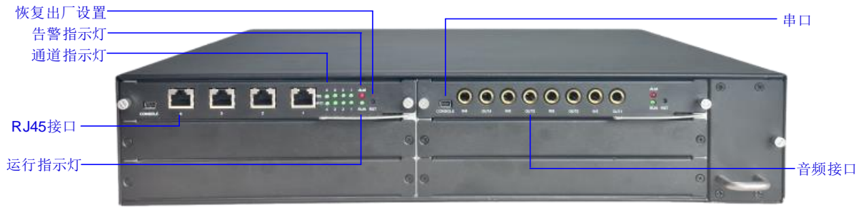
图 1-2 UNIWAY2300 前面板示意图
